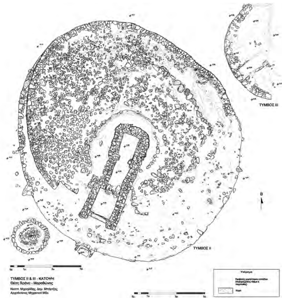
Σχ. 3. Κάτοψη τῶν Τύμβων II καὶ III στὴ σημερινή κατάσταση διατήρησης (2014, σχ. Ν. Μιχαηλίδη - Δ. Μπάρτζη).
