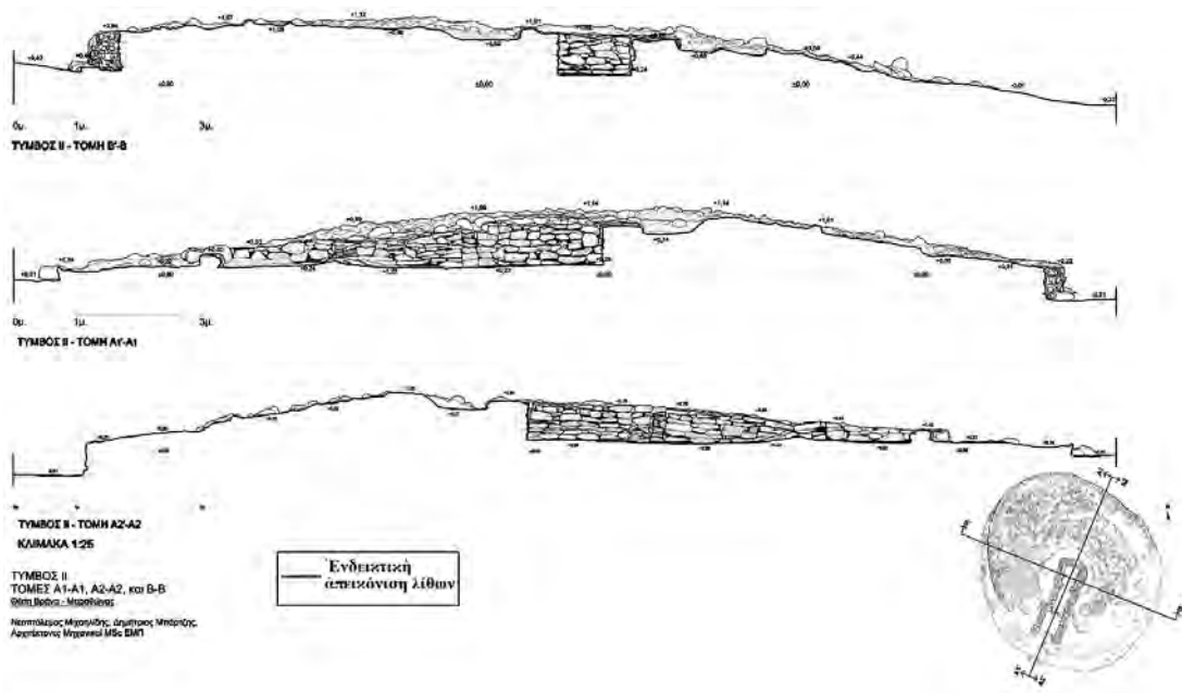
Σχ. 4. Σύγχρονες τομές του Τύμβου II (2014, σχ. Ν. Μιχαηλίδη - Δ. Μπάρτζη).
